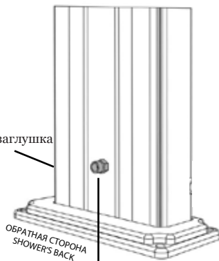
Подача воды 1/2" Water supply 1/2"
